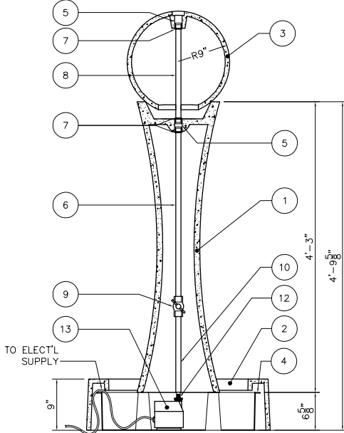
2 SECTION SCALE: 1/2"=1'
