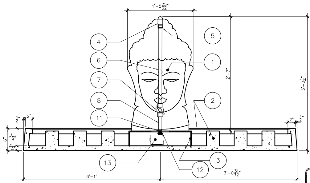
2 ELEVATION SCALE: 3/4"=1'-0"
